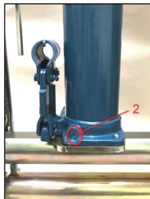
Pos. 2: Verschlusschraube (Weber-Hydraulik) bzw. roten Verschlussstopfen (Yale-Hydraulik) niemals entfernen oder Veränderungen vornehmen!
