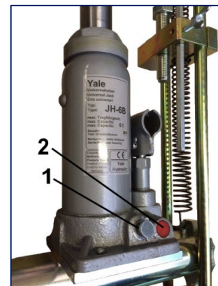
Pos. 2: Verschlusschraube (Weber-Hydraulik) bzw. roten Verschlussstopfen (Yale-Hydraulik) niemals entfernen oder Veränderungen vornehmen!
